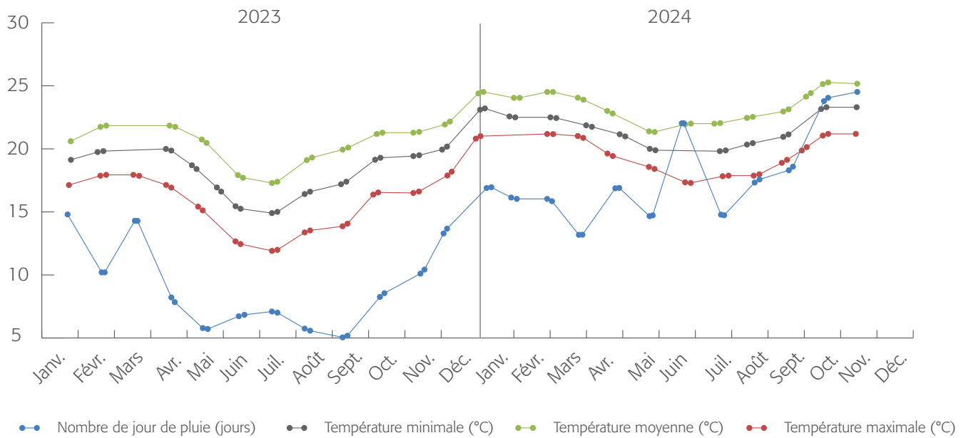
GRAPHIQUE N°2 : EVOLUTION DES INDICATEURS MÉTÉOROLOGIQUES DANS LA RÉGION ANALANJIROFO EN 2023 ET 2024
